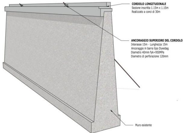
Vista prospettica del concio tipico di intervento Scala 1:---
