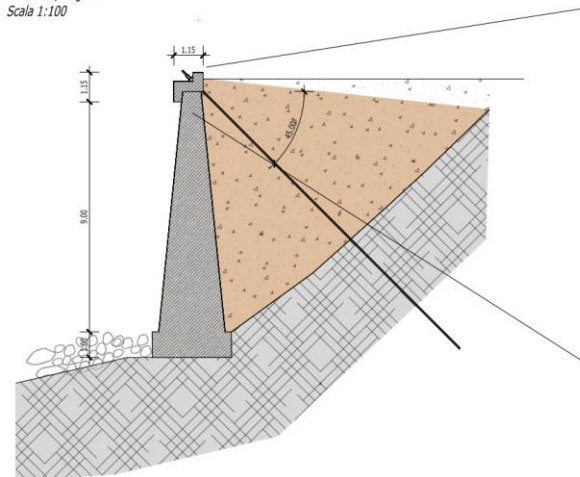
Sezione tipologica Scala 1:100
