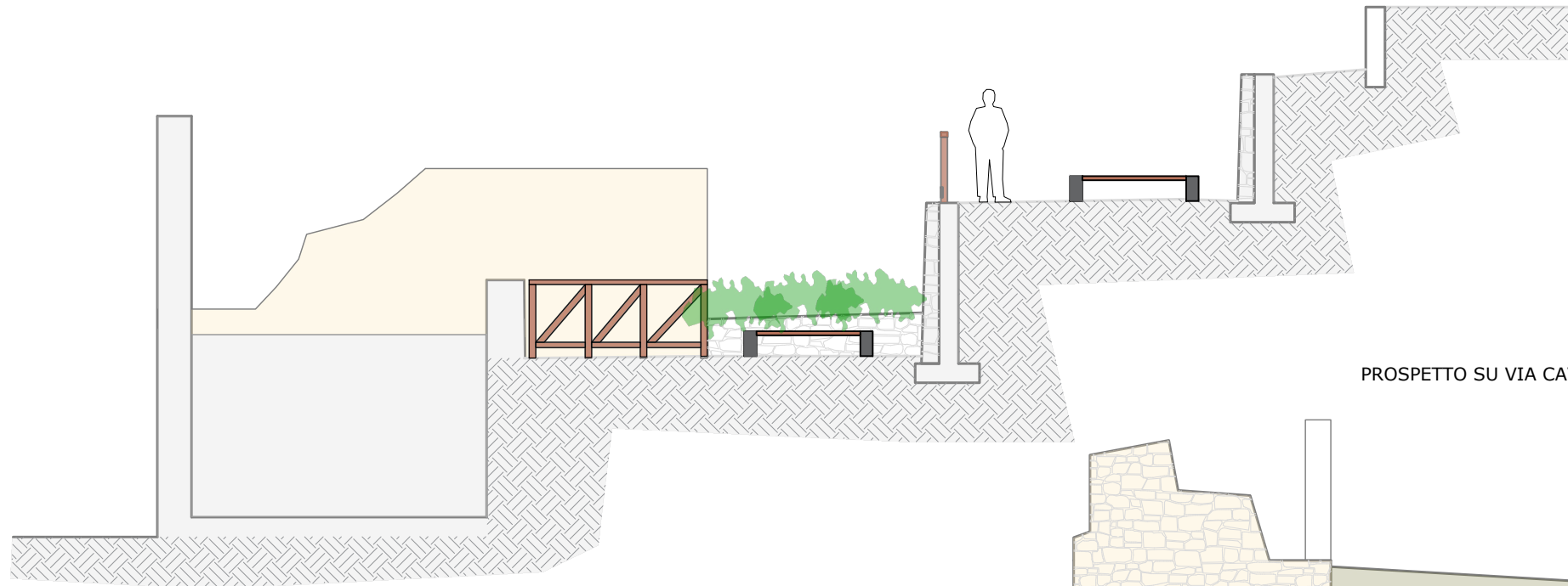
SEZIONE BB
