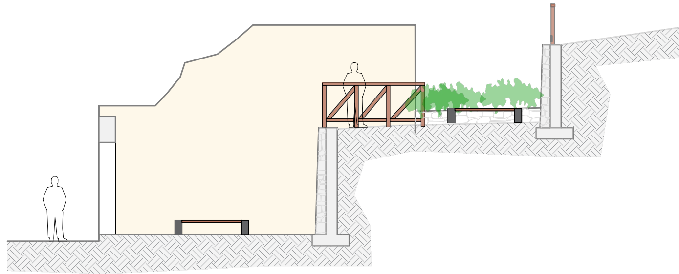
SEZIONE BB
