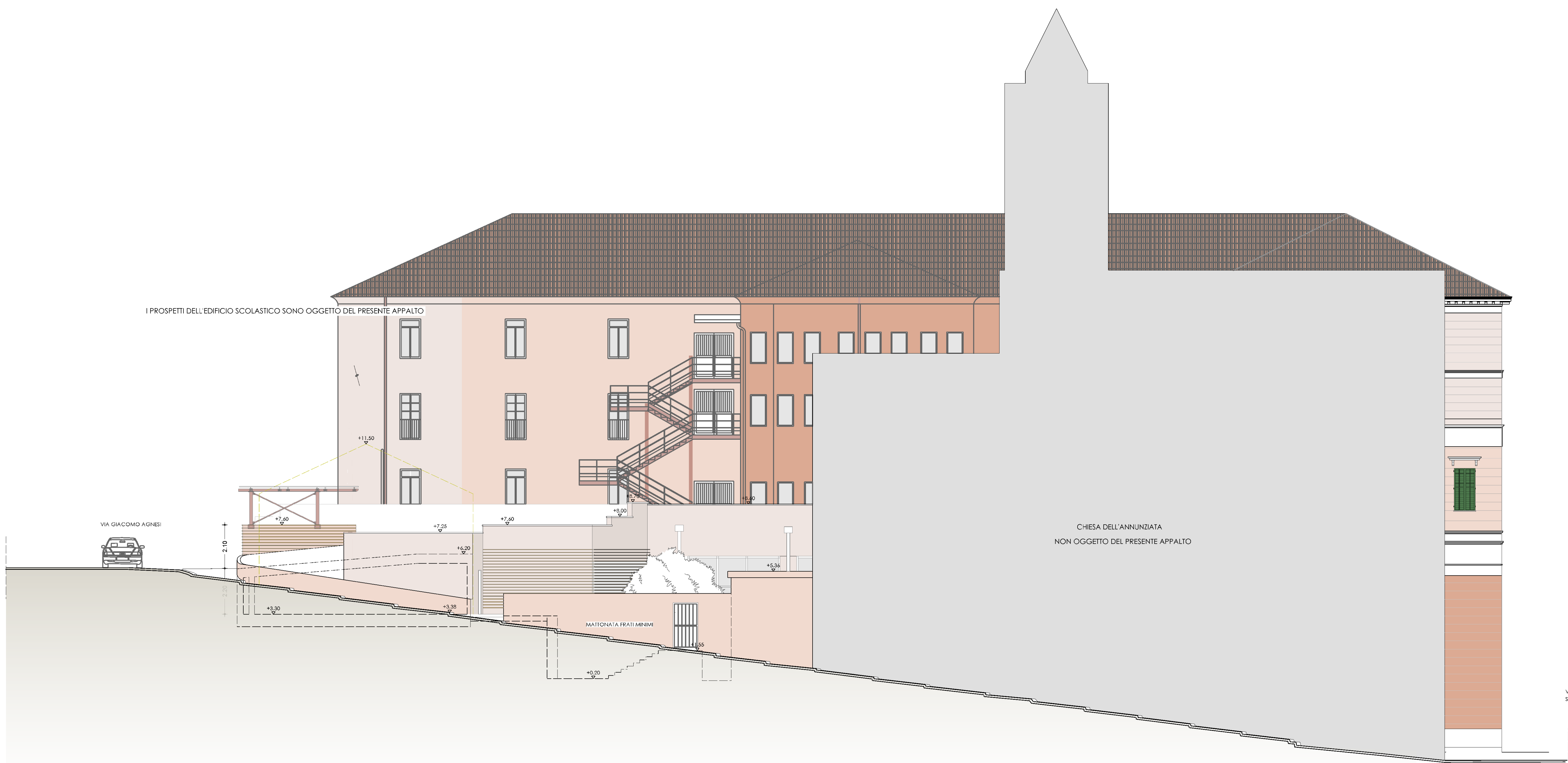
PROSPETTO OVEST
