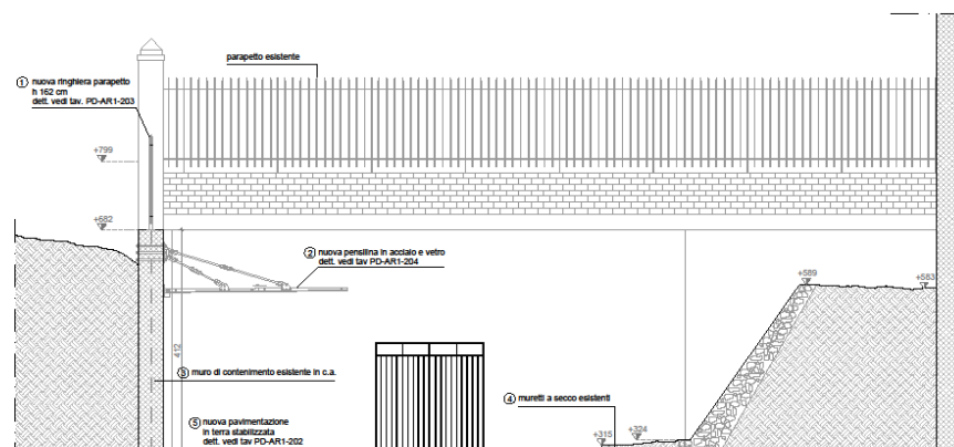
SEZIONE 4 scala 1:50
