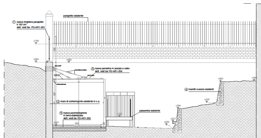
SEZIONE 4 scala 1:50
